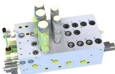
土方设备控制阀块 (二型)
